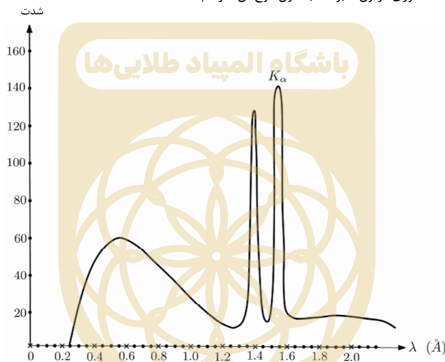
شکل ۱: شدت فوتون‌های آشکار شده برحسب طول موج
