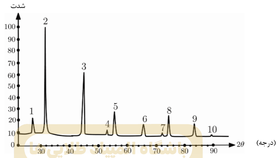
شکل ۴: پراش پرتوهای ایکس از دسته صفحات براگ مختلف بلور نمک
